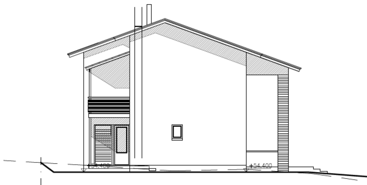
JULKISIVU LUOTEESEEN
