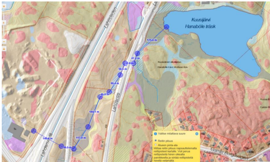
Kuva 6. Haxlogin tontin hulevesien pumppaus ja virtausreitti Kuusijärveen (l=990 m)
