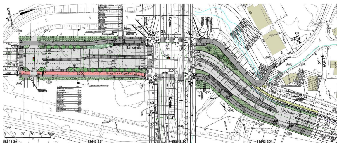
Kuva 22. Lahdentie – Kyytitien risteyksen katusuunnitelmaluonnos (Finnmap Infra, luonnos 9.3.2022).
