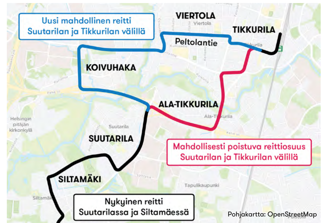
Kuva 4.27 Linjan 611 nykyinen reitti ja mahdollinen reittimuutos Suutarilan ja Tikkurilan välillä.
