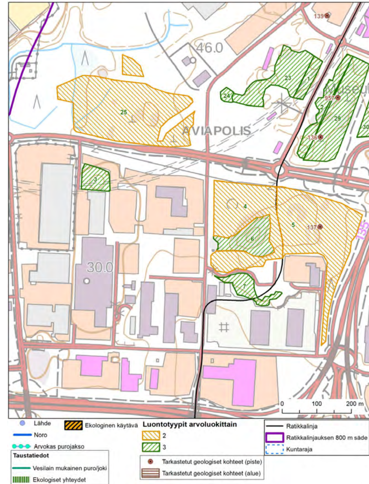
Kuva 6.22 Arvokkaat luontokohteet ja tarkastetut geologiset kohteet Aviapolisen alueella. (Lähde: Vantaan ratikan kaavarunkoalueen luontoselvitykset 2020–2021 Koosteraportti, Faunatica 2021).
