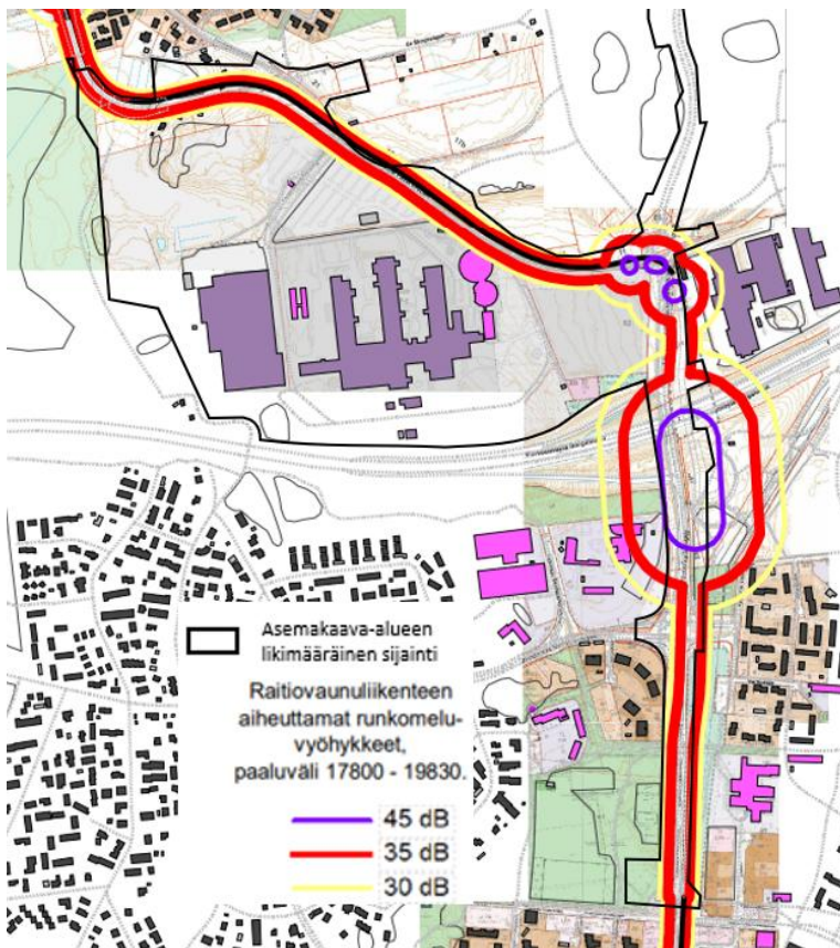
Kuva 43. Raitiovaunuliikenteen aiheuttamat runkomelualueet Vaaralan eteläosassa ja Länsimäen pohjoisosissa, paaluväli 16000–18300 (Täriä- ja runkomeluselvitys, WSP Finland Oy ja Afry Finland Oy, 18.1.2023).
