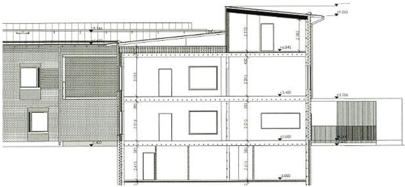
Leikkaus A-A.
