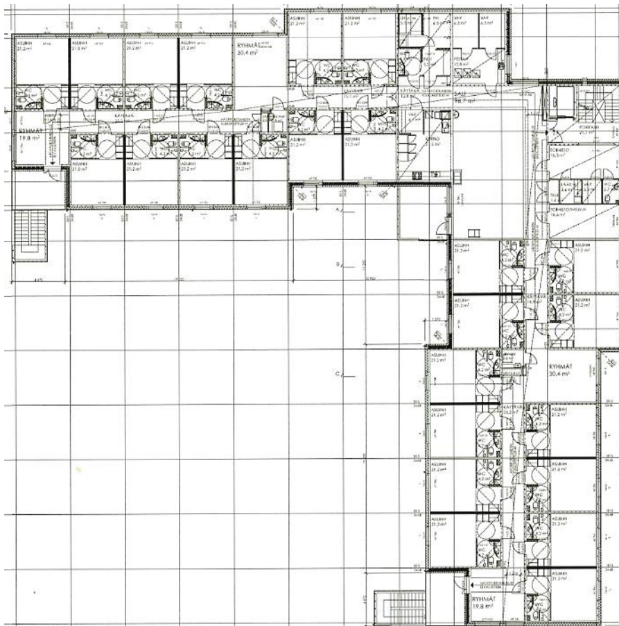
2. kerros.
