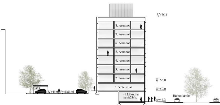
Leikkaus aa
