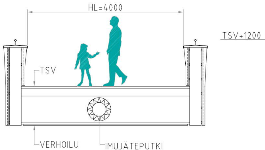
Sillan periaatepoikkileikkaus
