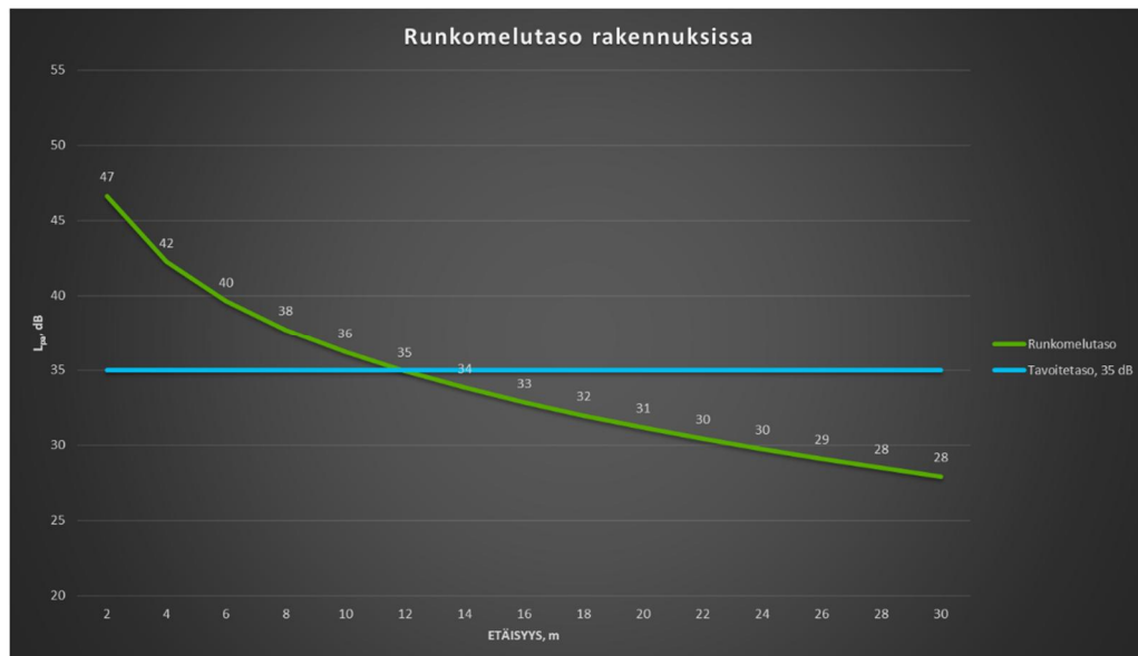
Kuva 7. Runkomelutaso rakennuksissa
