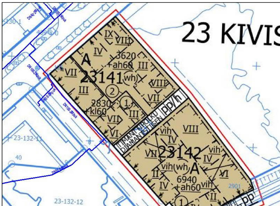
Kaukolämpöverkko asemakaavaehdotuskartalla
