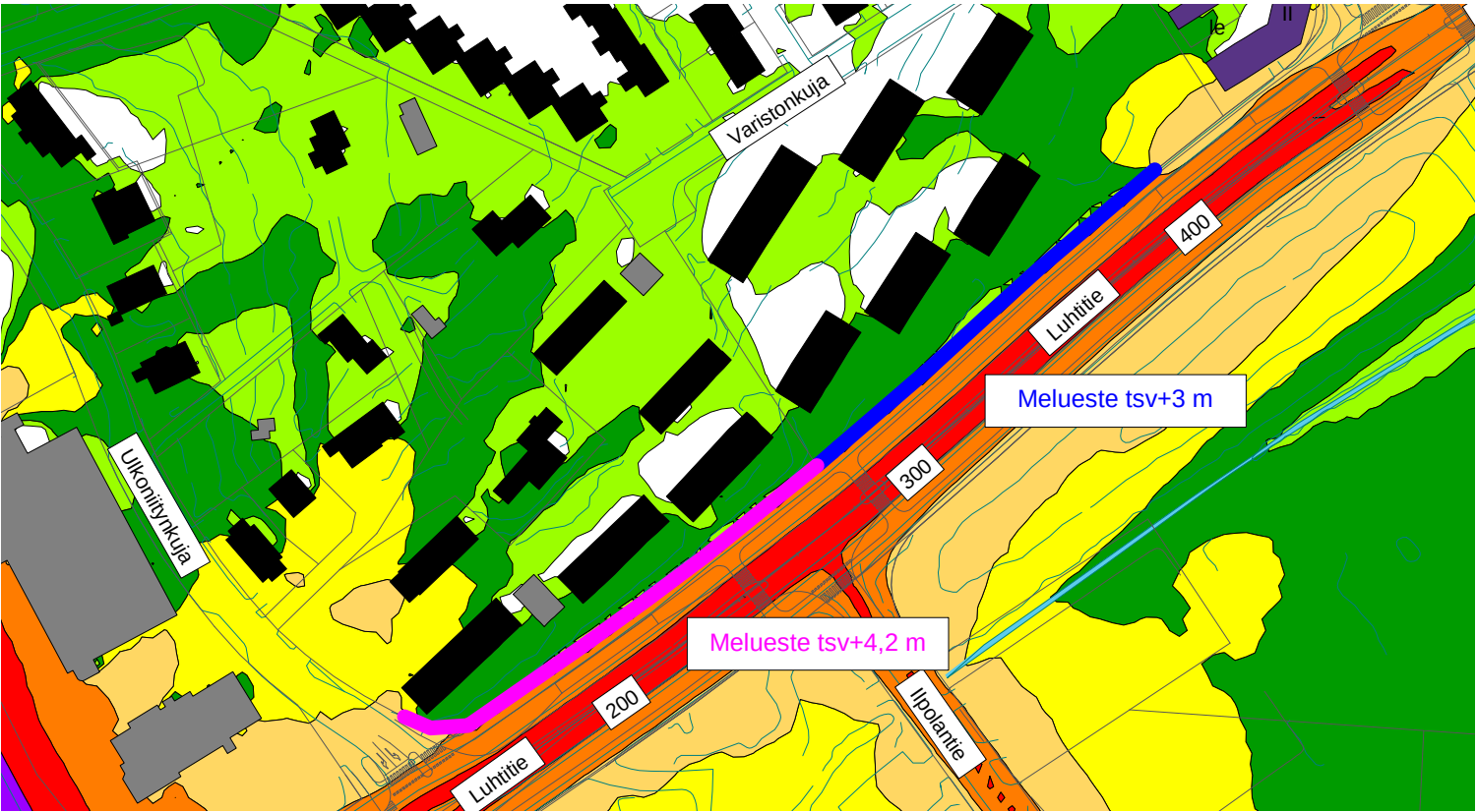
Melueste korkeampi Ulkonäytinkujan rakennusten kohdalla, esteessä ei kulkuaukkoja tai ne on toteutettu ovina tai limitettyinä.
