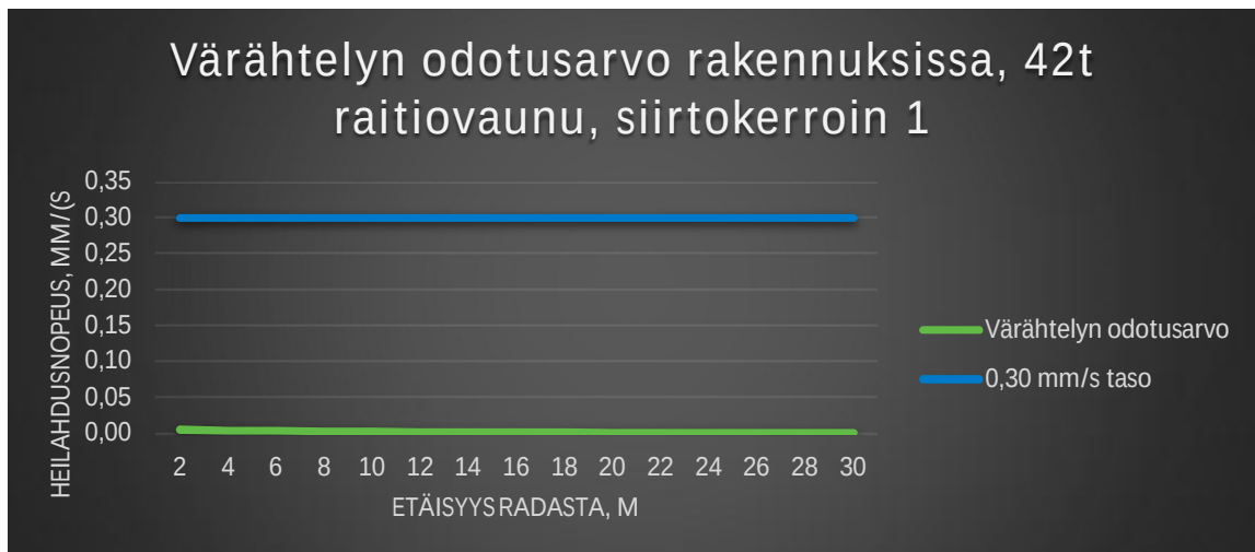
Kuva 6. Tärinän leviämislaskennan tulokset maaperän ollessa kalliota.
