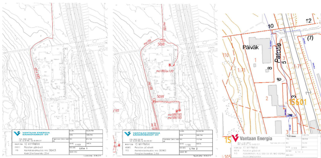
Keskijänniteverkon kartta
