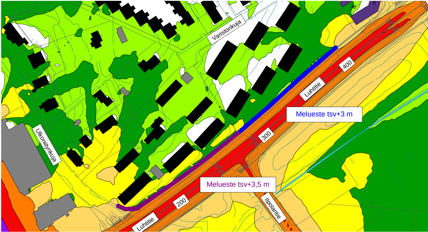
Melueste korkeampi Ulkonäytinkujan rakennusten kohdalla, esteessä 2 m leveät kulkuaukot.
