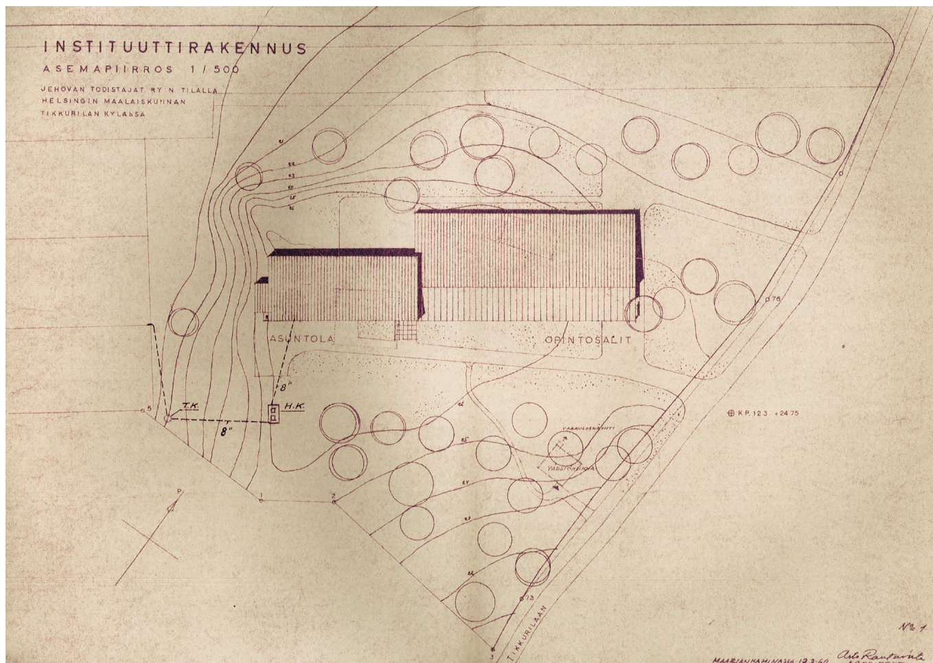
Asuin- ja koulutusrakennuksen asemapiirros vuodelta 1960 (Vantaan kaupunginmuseo).
