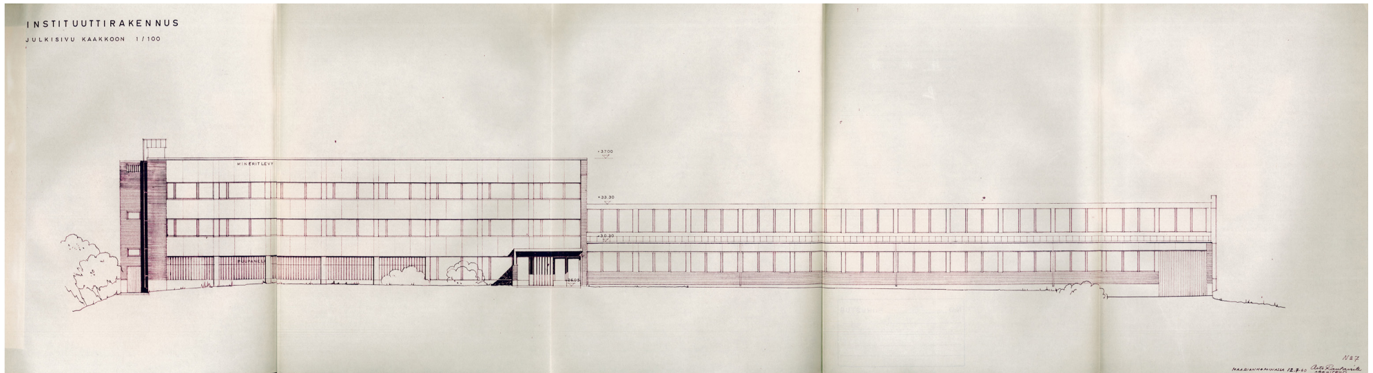
Asuin- ja koulutusrakennuksen kaakkaisjulkisivu vuodelta 1960 (Vantaan kaupunginmuseo).
