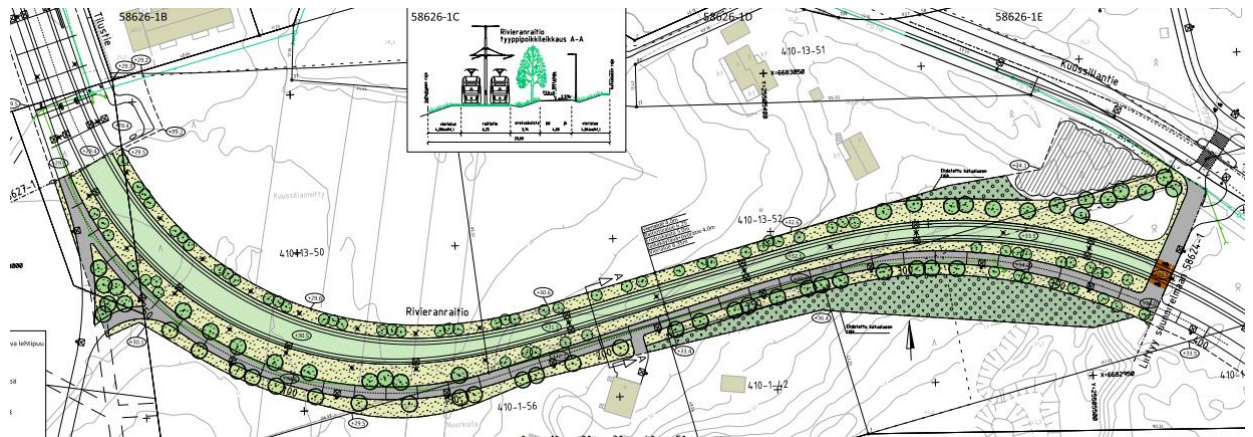
Kuva 29. Katusuunnitelmaluonnos Rivieranraitilta (AFRY Finland Oy, luonnos 7.10.2021).
