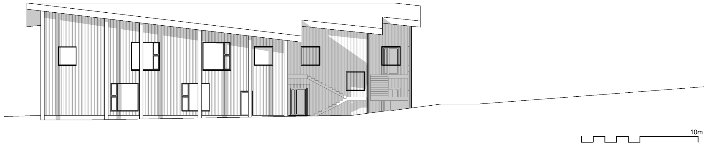
Julkisivu koilliseen 1 : 200
