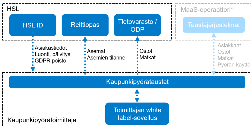
Kuva 10. Vaiheen 1 arkkitehtuuri (HSL).
