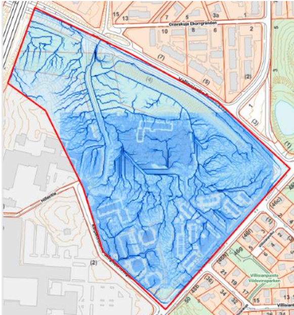
Virtauskertymä ja kosteusindeksi kaavamuuotosalueella ja sen eteläpuolisissa kortteleissa. Vantaan kaupungin valuma-alueyökalu.
