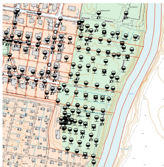
Pohjatutkimuspisteet.
