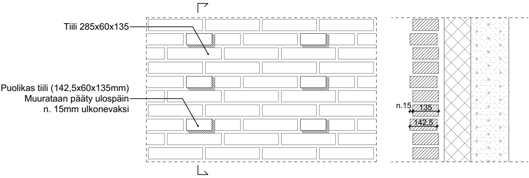
DETALJIOTE tehostemuuraus
