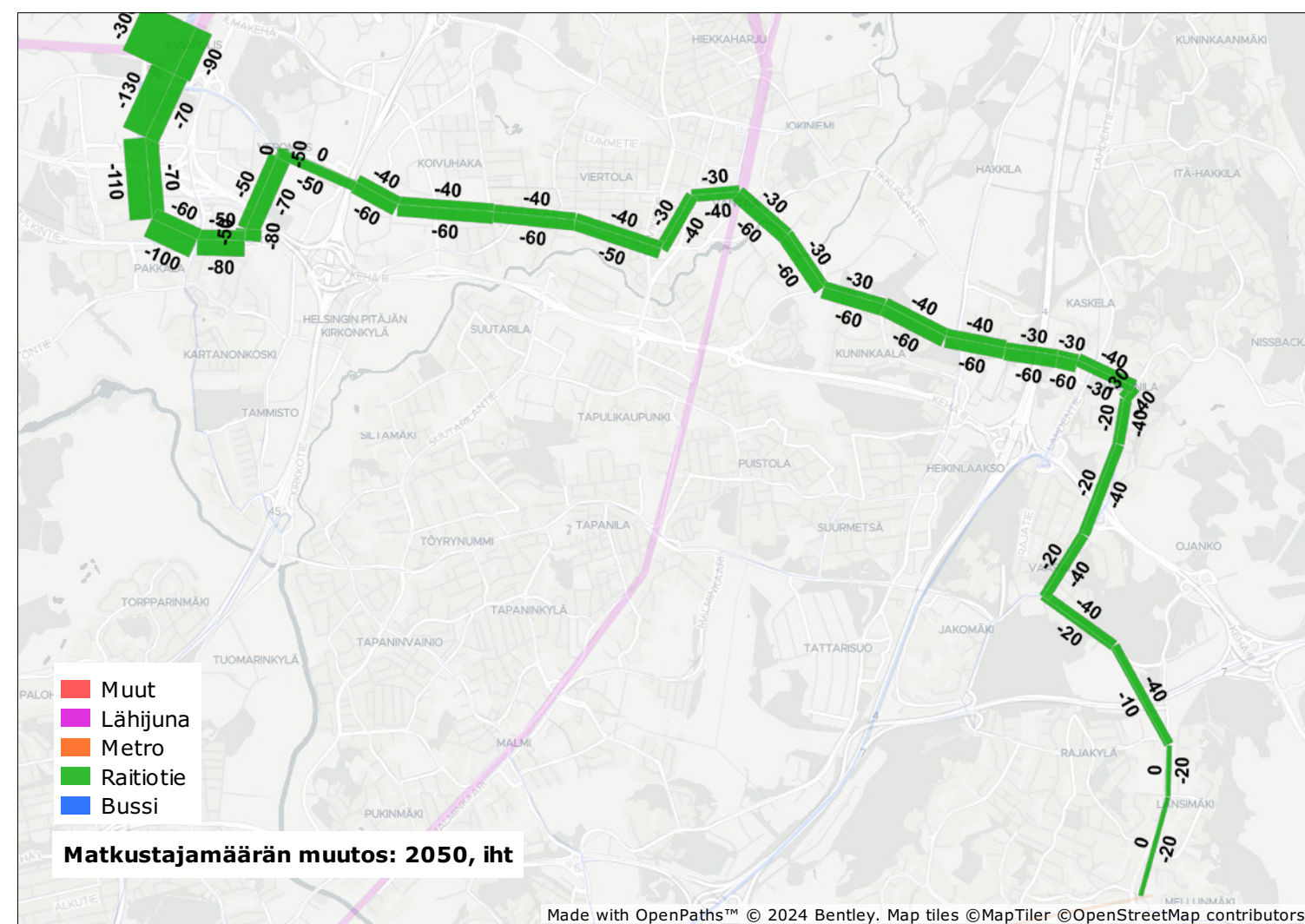
Kuva 3.4 Ennustettu matkustajamäärien muutos iltahuipputunnille vuonna 2050 verrattuna hankesuunnitelmaan 2023.
