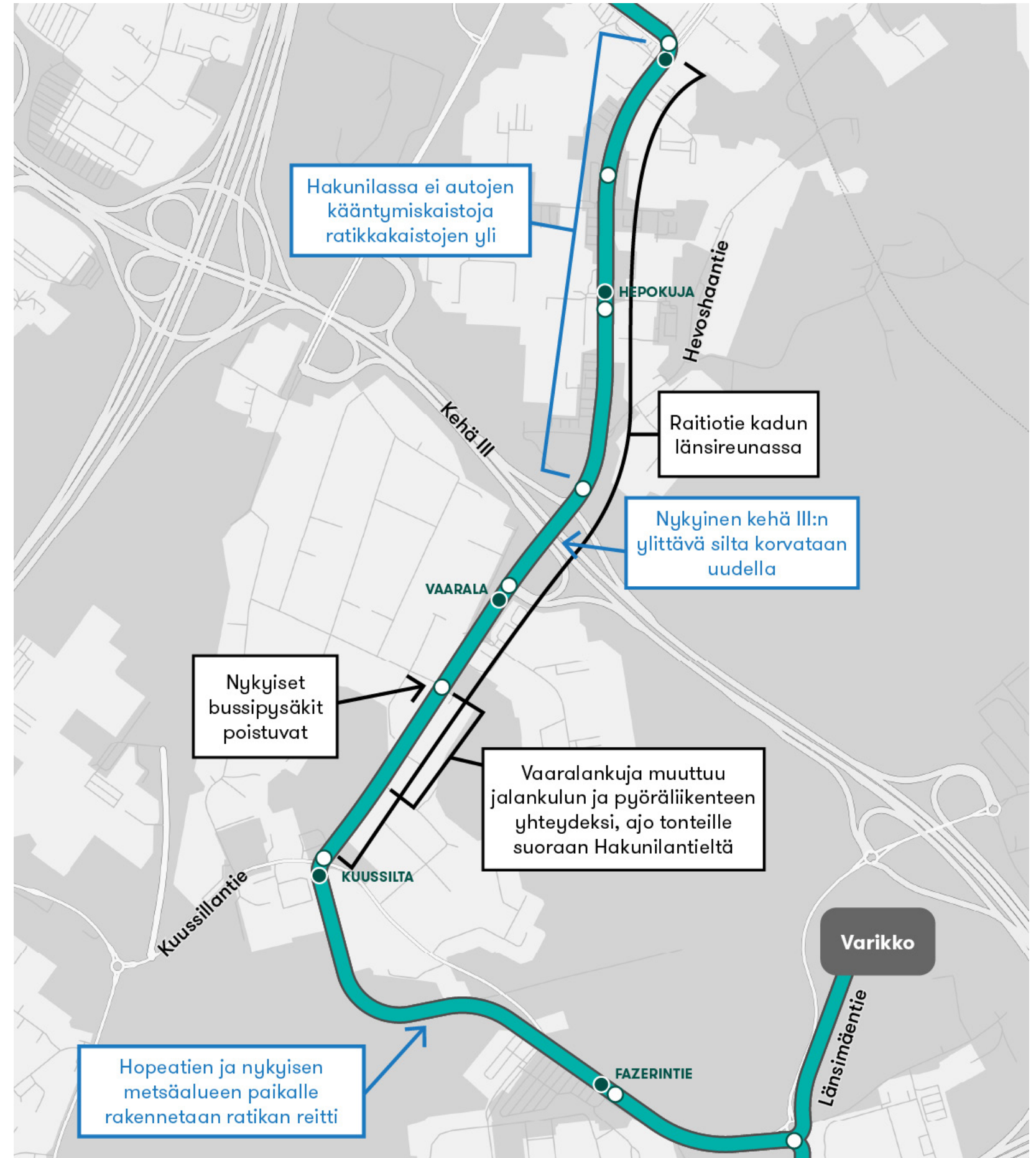
Kuva 2.25 Joukkoliikenteen ja autoliikenteen yhteydet ja muutokset vuoden 2023 hanksuunnitelmaan Hakunilantiella ja Fazerintieellä.
