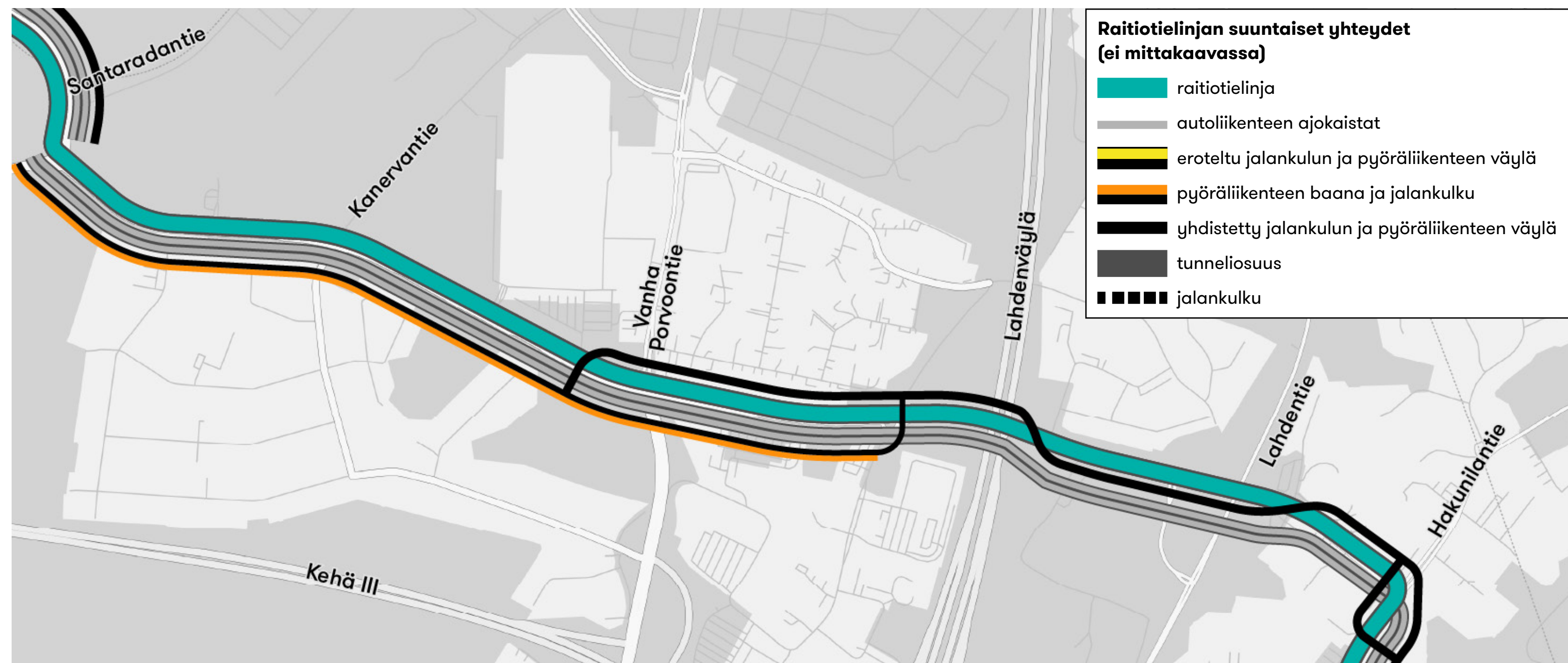
Kuva 2.19 Raitiotielinjan suuntaiset yhteydet Kyytitiellä.
