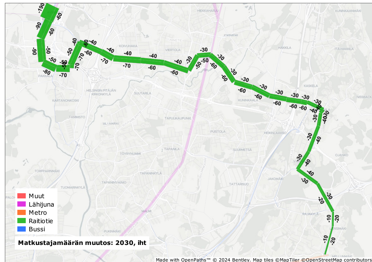
Kuva 3.2 Ennustettu matkustajamäärien muutos iltahuipputunnille vuonna 2030 verrattuna hankesuunnitelmaan 2023.
