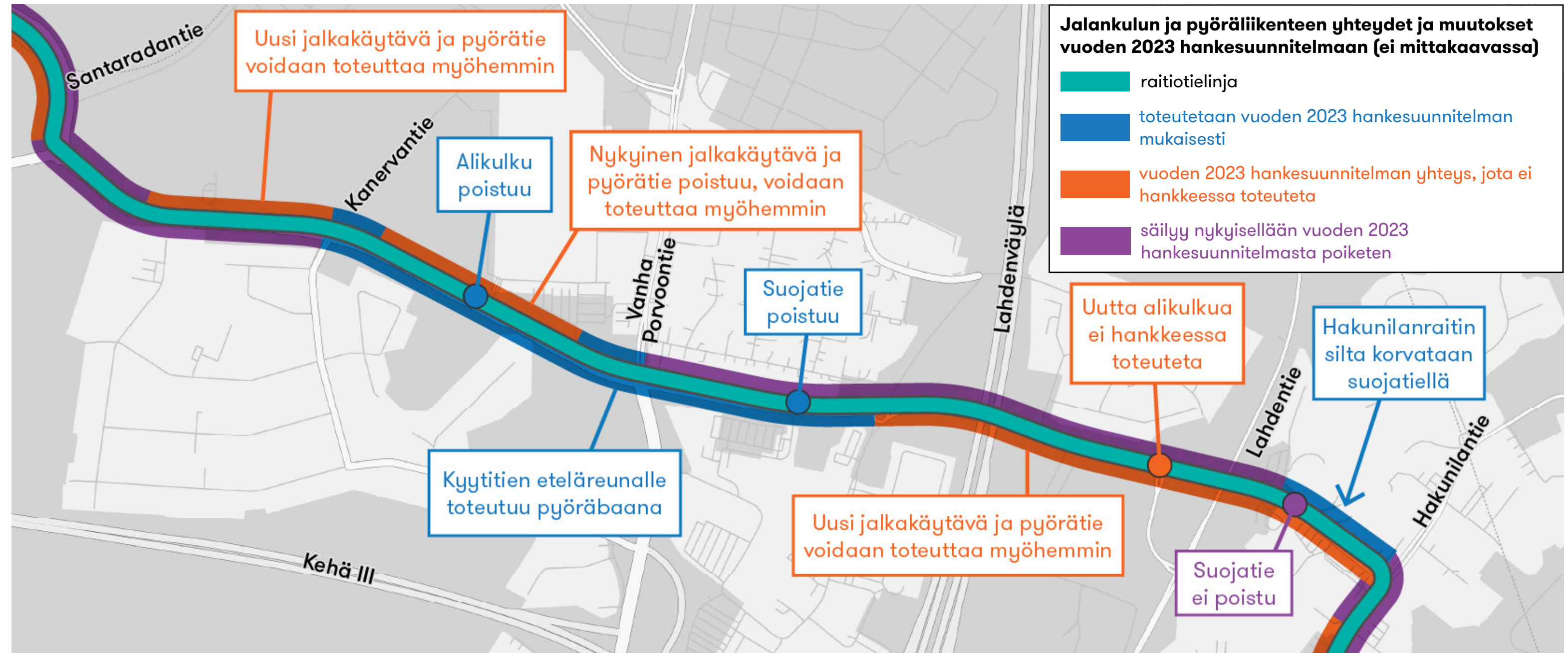
Kuva 2.20 Jalankulun ja pyöräliikenteen yhteydet ja muutokset vuoden 2023 hankesuunnitelmaan Kyytitiellä.
