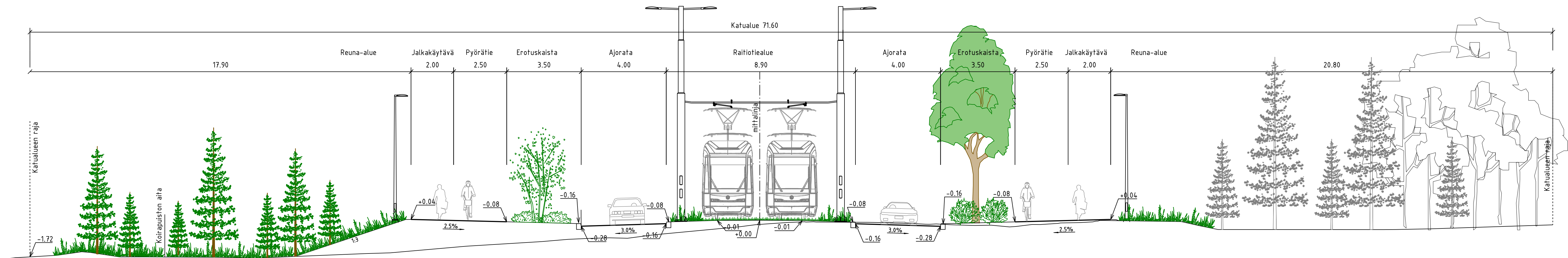
TYYPPIPOIKKILEIKKAUS A-A
