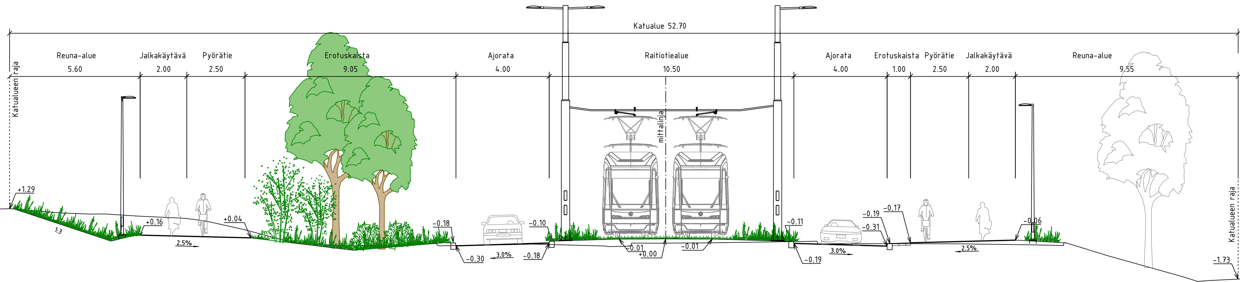
TYYPPIPOIKKILEIKKAUS C-C
