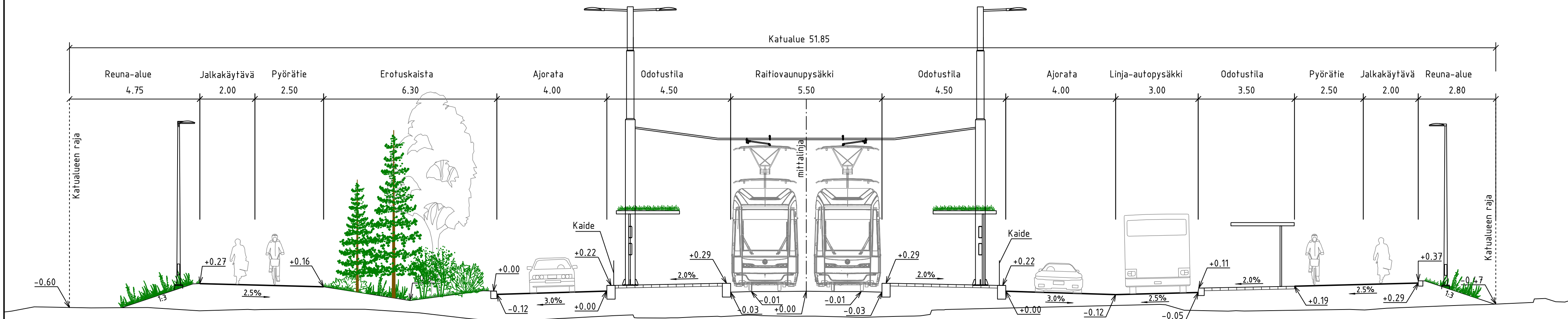
TYYPPIPOIKKILEIKKAUS B-B
