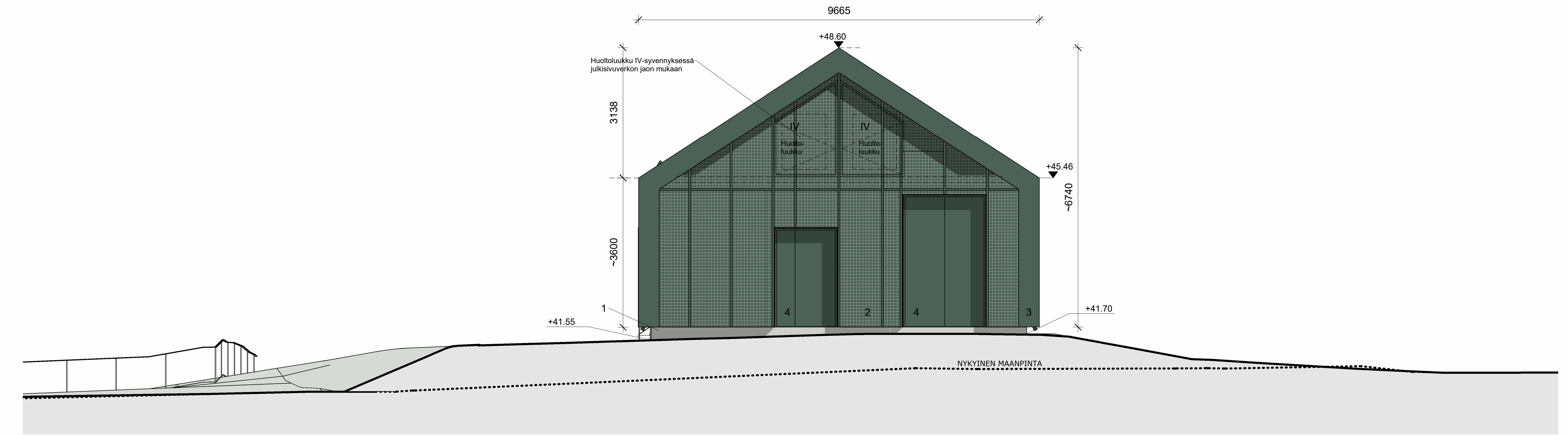
JULKISIVU POHJOISEEN 1 : 50
