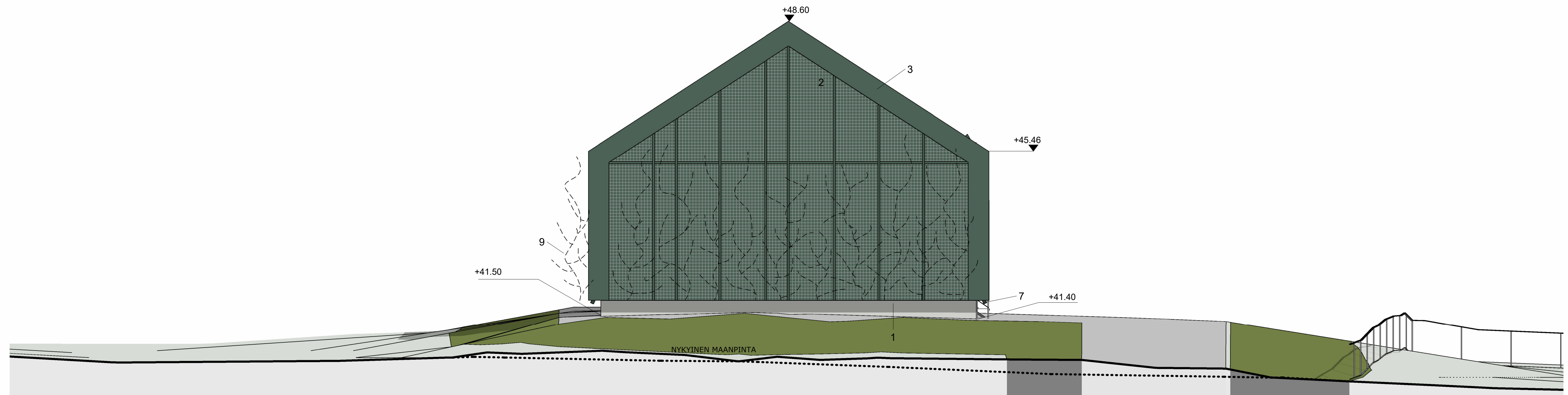
JULKISIVU ETELÄÄN 1 : 50
