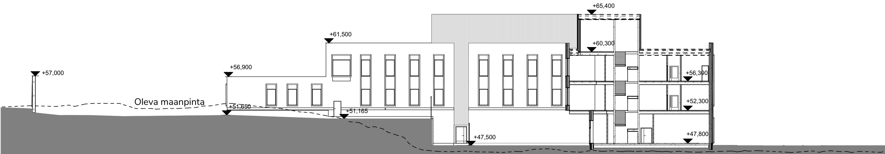
2. ALUELEIKKAUS 1:300
