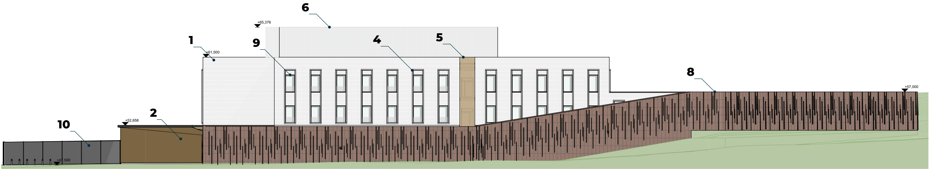
1 JULKISIVU LUOTEeseen 1:300
