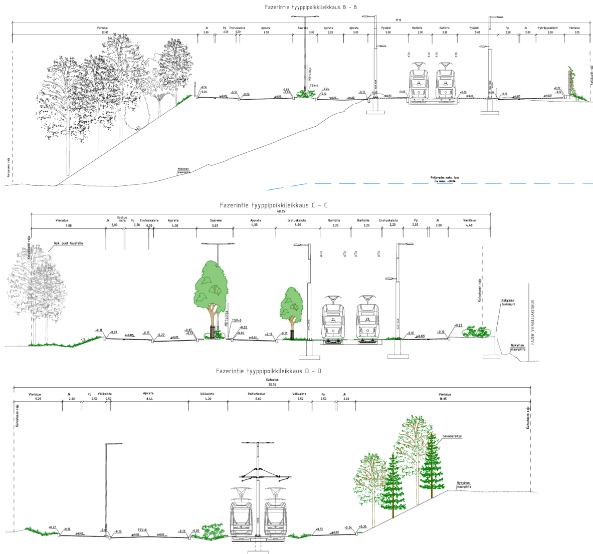
Kuvat 34-36. Tyypipiikkileikkaukset Fazerintiellä. (Sweco Finland, luonnos 26.1.2026)
