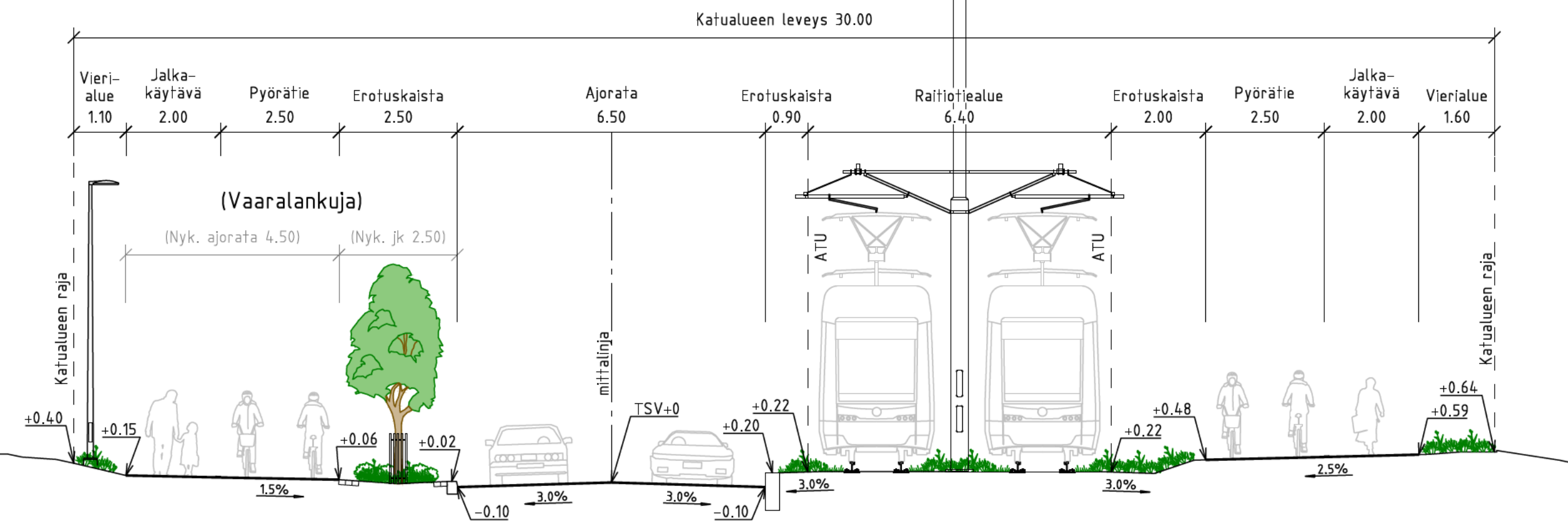
TYYPPIPOIKKILEIKKAUS A-A Hakunilantie välillä Vaaralan talkootie - Kirkkokuja
