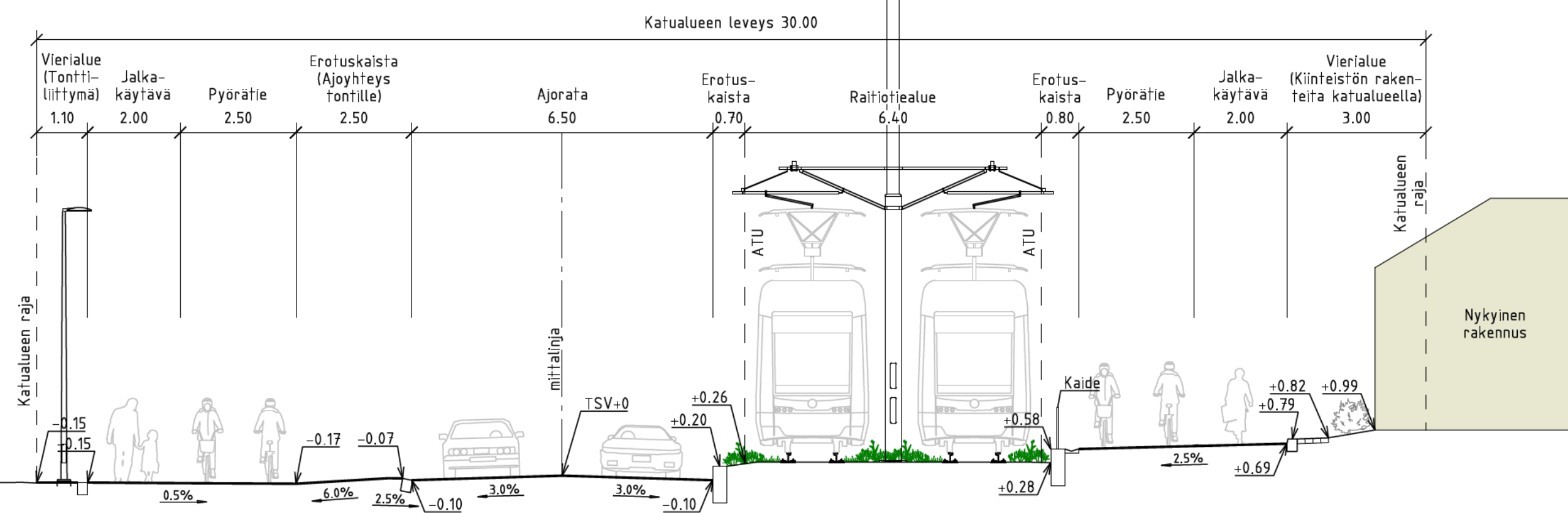
TYYPPIPOIKKILEIKKAUS B-B Hakunilantie välillä Vaaralan talkootie - Kirkkokuja
