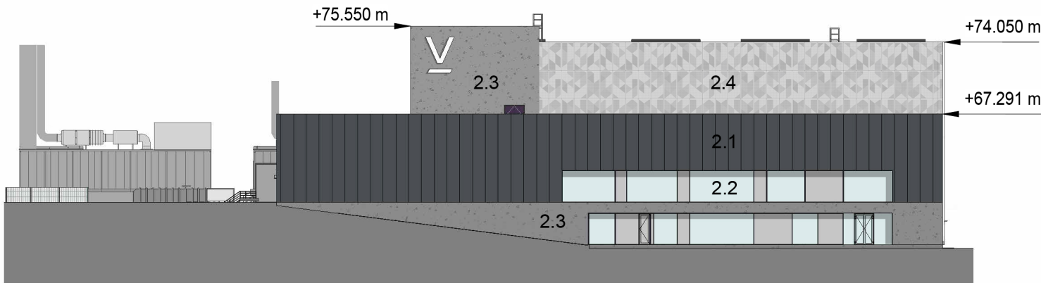
Julkisivu itään 1:500
