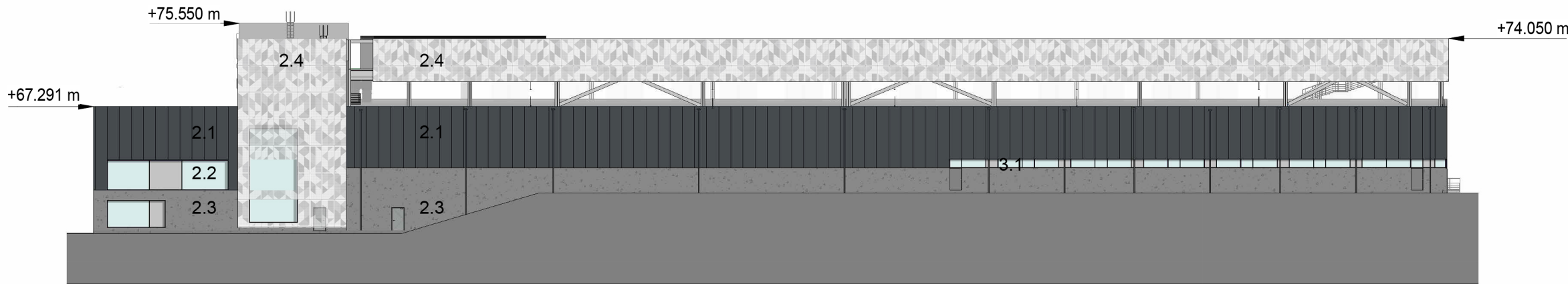
Julkisivu pohjoiseen 1:500
