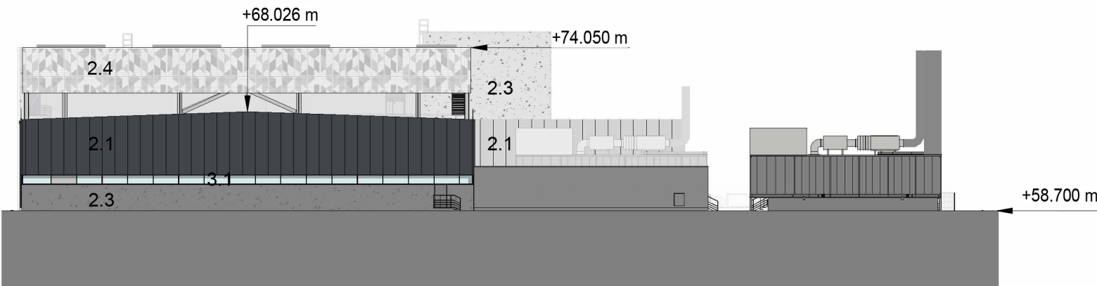
Julkisivu länteen 1:500
